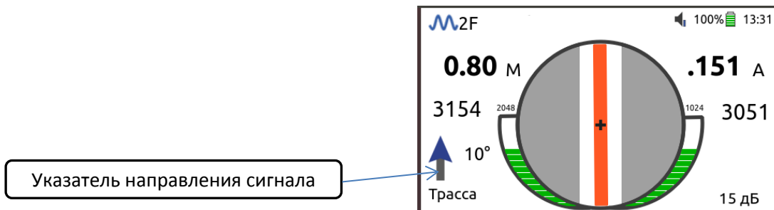
Рисунок 3.18. Указатель направления сигнала в режиме «2F».
