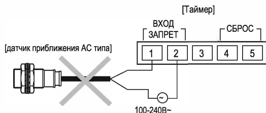
< Неправильное соединение >
