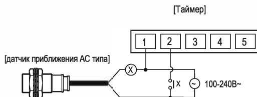
< Правильное соединение >
