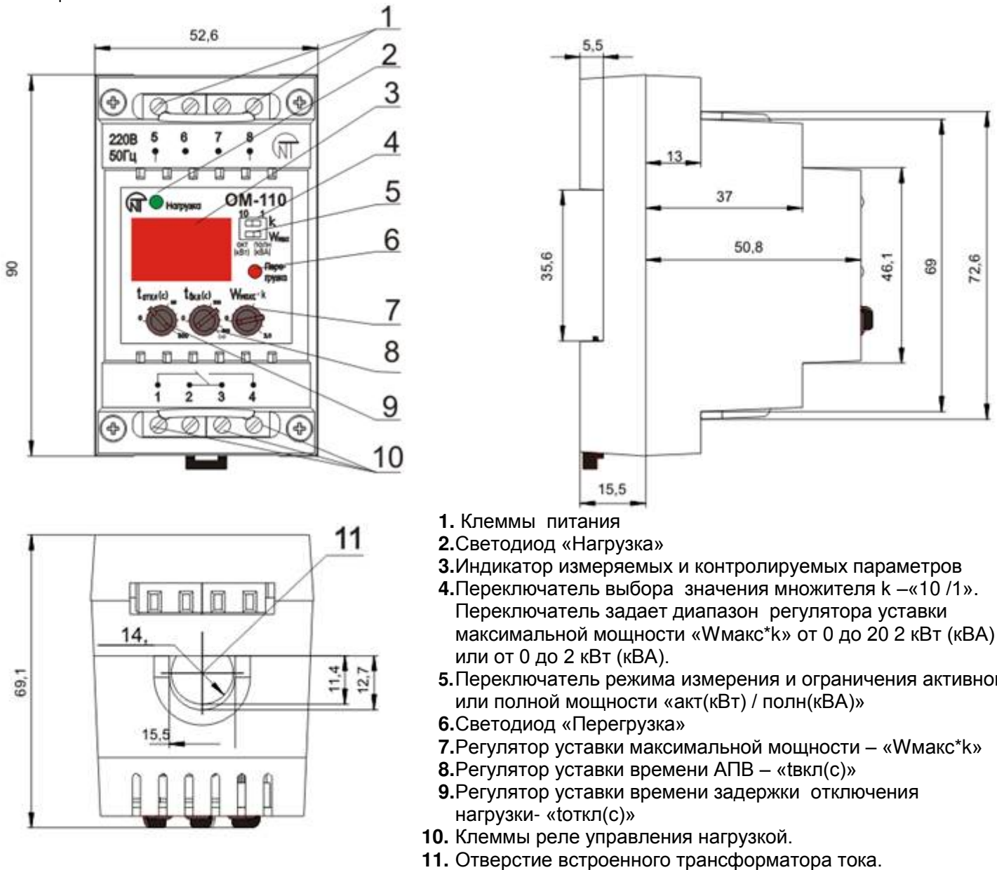
Рисунок 1- Внешний вид ОМ-110-01
