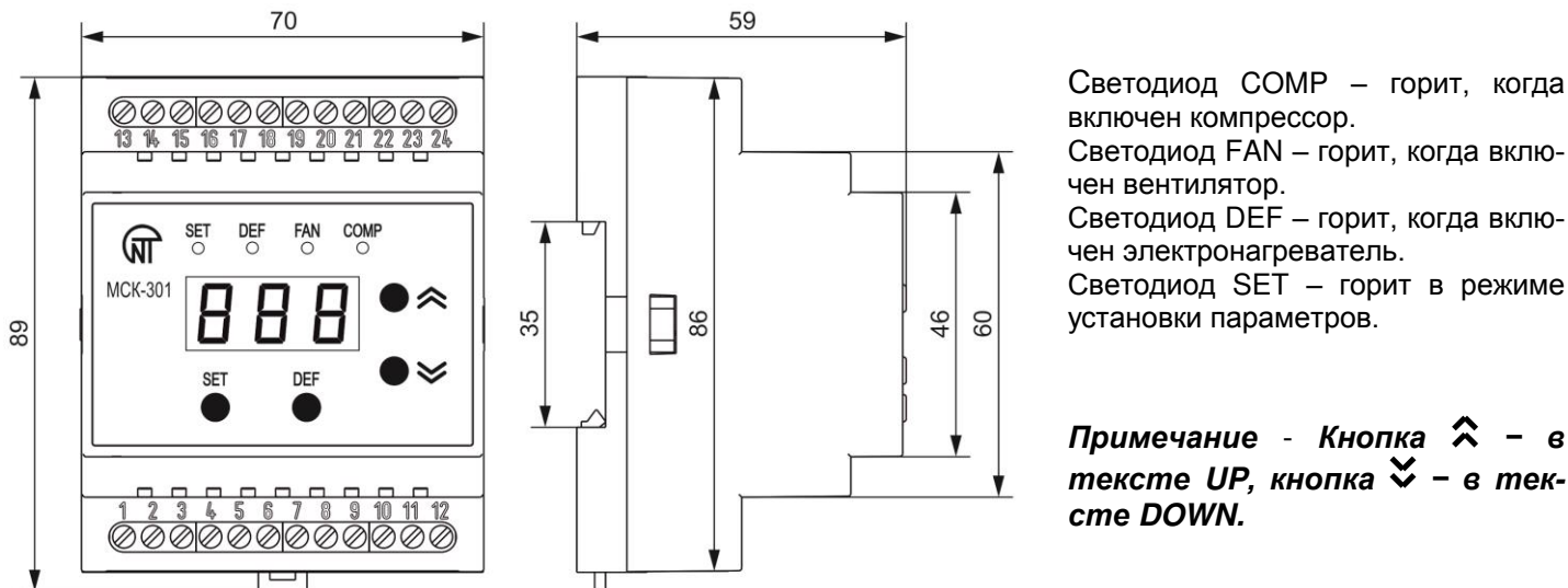
Рисунок 1 – Лицевая панель, органы управления и габаритные размеры МСК-301-54
