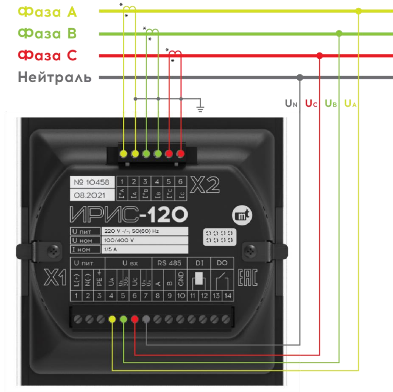
Рисунок 10.1 - Схема подключения устройства с внешними трансформаторами тока, без трансформаторов напряжения (ЗТ, 0ТН)
