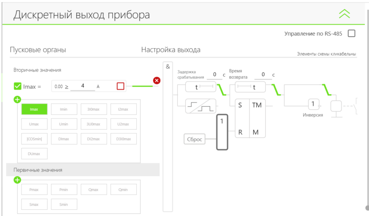
Рисунок 4.2 - Алгоритм работы дискретного выхода
