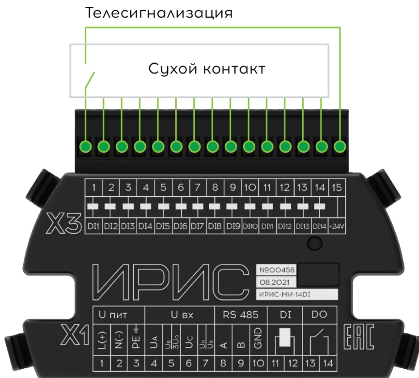
Рисунок 12.5 - Схема подключения рюкзак ИРИС - 14DI
