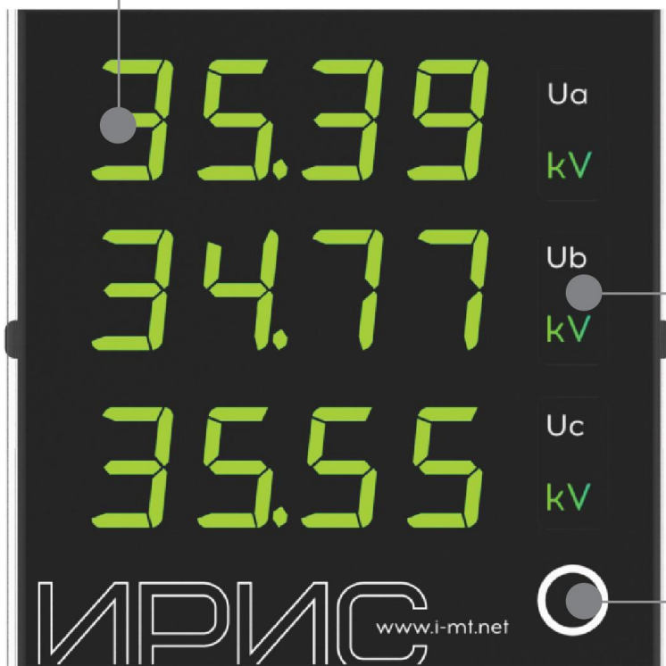
Рисунок.3.3 - Внешний вид лицевой панели ИРИС
