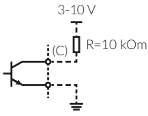
Схема подключения импульсного кабеля
