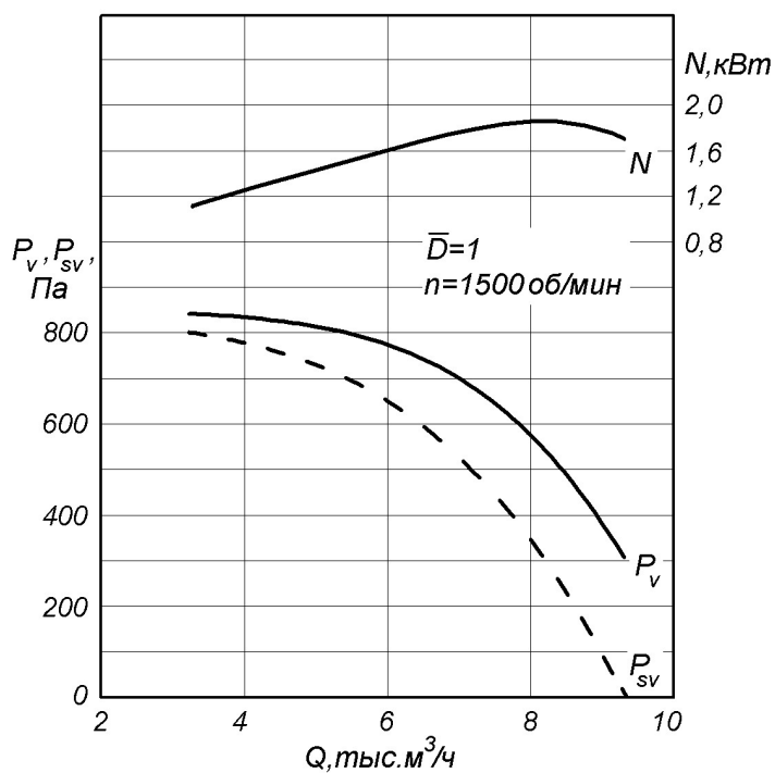
РАДИВЕЙ®-...-11-5 ( n = 1500 об/мин) D = D_{\text{ном}}
