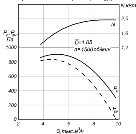
РАДИВЕЙ®-...-11-5 ( n = 1500 об/мин) D = 1,05 D_{\text{ном}}
