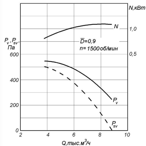
РАДИВЕЙ®-...-11-5 ( n = 1500 об/мин) D = 0,9 D_{\text{ном}}
