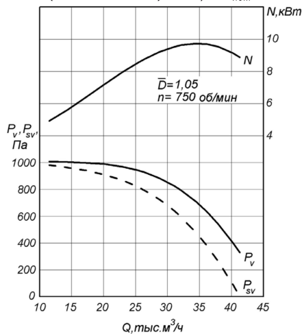
РАДИВЕЙ®-...-11-10 ( n = 750 об/мин) D = 1,05 D_{\text{ном}}
