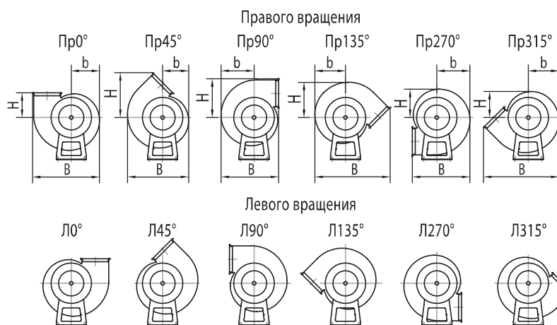
Положения корпуса вентилятора
