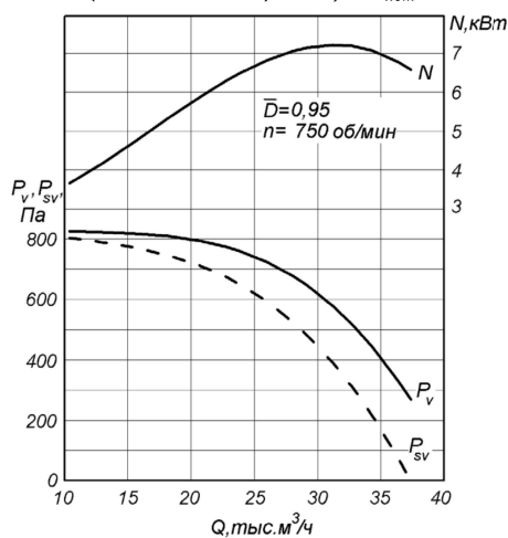
РАДИВЕЙ®-...-11-10 ( n = 750 об/мин) D = 0,95 D_{\text{ном}}
