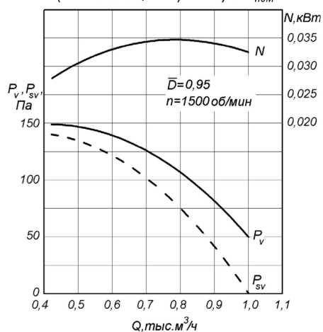
РАДИВЕЙ®-...-11-2,5 ( n = 1500 об/мин) D = 0,95 D_{\text{ном}}
