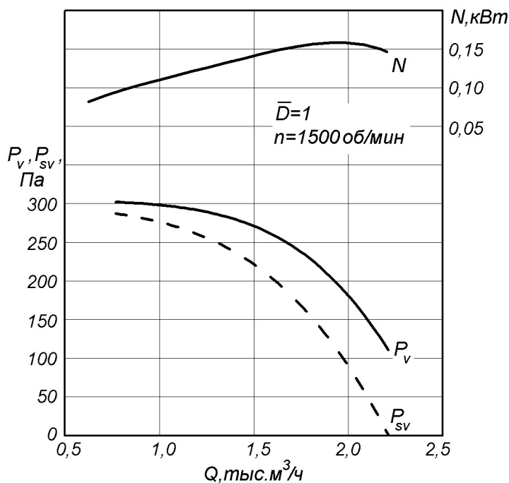
РАДИВЕЙ®-...-11-3,15 ( n = 1500 об/мин) D = D_{\text{НОМ}}
