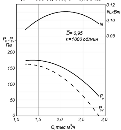
РАДИВЕЙ®-...-11-4 ( n = 1000 об/мин) D = 0,95 D_{\text{НОМ}}
