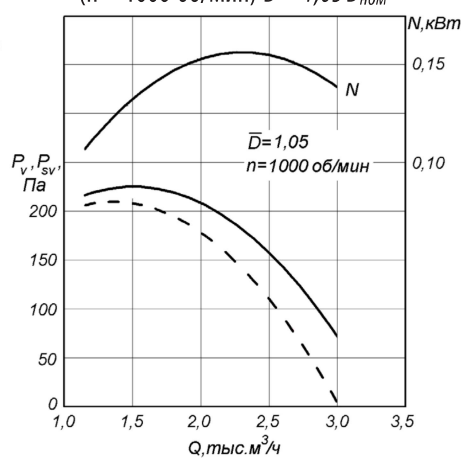
РАДИВЕЙ®-...-11-4 ( n = 1000 об/мин) D = 1,05 D_{\text{НОМ}}
