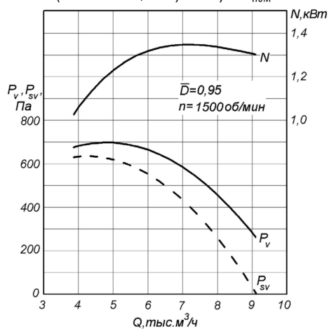
РАДИВЕЙ®-...-11-5 ( n = 1500 об/мин) D = 0,95 D_{\text{ном}}
