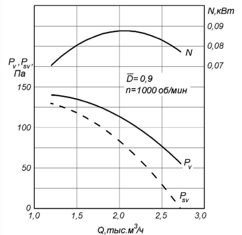
РАДИВЕЙ®-...-11-4 ( n = 1000 об/мин) D = 0,9 D_{\text{НОМ}}
