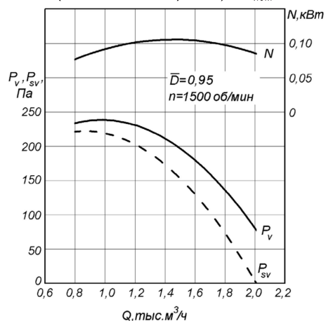
РАДИВЕЙ®-...-11-3,15 ( n = 1500 об/мин) D = 0,95 D_{\text{НОМ}}
