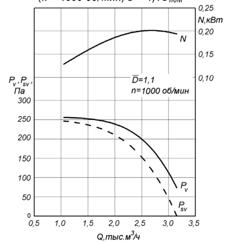
РАДИВЕЙ®-...-11-4 ( n = 1000 об/мин) D = 1,1 D_{\text{НОМ}}
