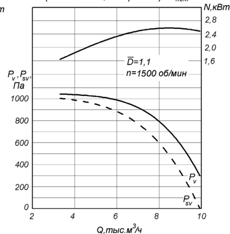
РАДИВЕЙ®-...-11-5 ( n = 1500 об/мин) D = 1,1 D_{\text{ном}}
