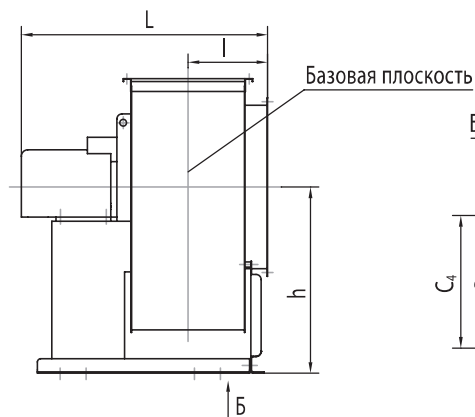
Положения корпуса вентилятора
