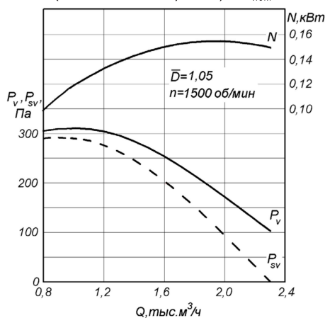
РАДИВЕЙ®-...-11-3,15 ( n = 1500 об/мин) D = 1,05 D_{\text{НОМ}}
