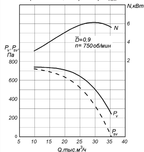
РАДИВЕЙ®-...-11-10 ( n = 750 об/мин) D = 0,9 D_{\text{ном}}
