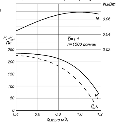
РАДИВЕЙ®-...-11-2,5 ( n = 1500 об/мин) D = 1,1 D_{\text{ном}}
