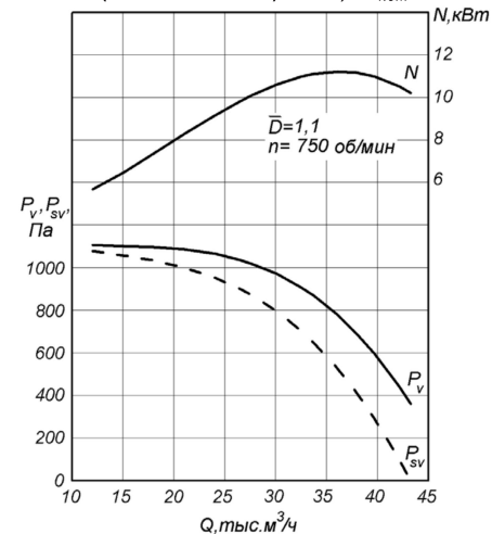
РАДИВЕЙ®-...-11-10 ( n = 750 об/мин) D = 1,1 D_{\text{ном}}
