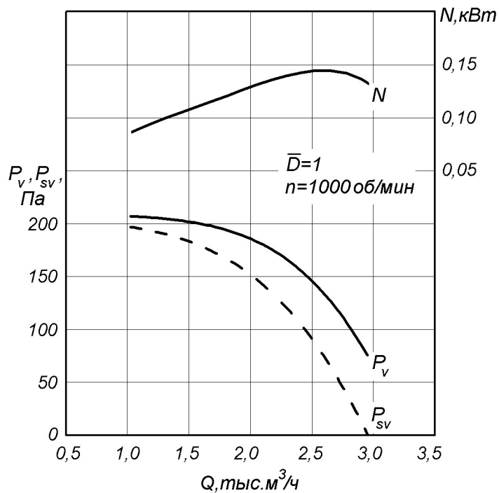
РАДИВЕЙ®-...-11-4 ( n = 1000 об/мин) D = D_{\text{НОМ}}
