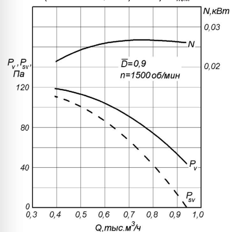
РАДИВЕЙ®-...-11-2,5 ( n = 1500 об/мин) D = 0,9 D_{\text{ном}}
