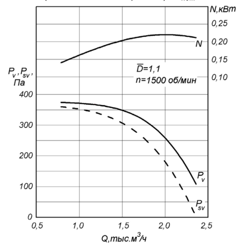
РАДИВЕЙ®-...-11-3,15 ( n = 1500 об/мин) D = 1,1 D_{\text{НОМ}}
