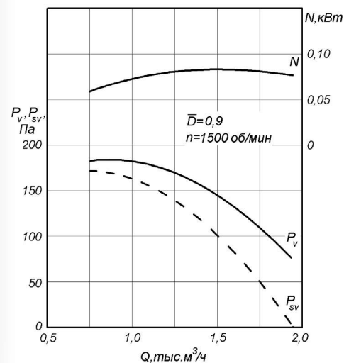
РАДИВЕЙ®-...-11-3,15 ( n = 1500 об/мин) D = 0,9 D_{\text{НОМ}}
