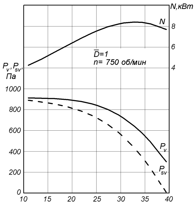
РАДИВЕЙ®-...-11-10 ( n = 750 об/мин) D = D_{\text{ном}}
