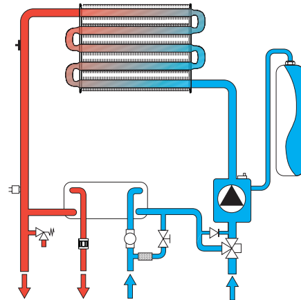
ГИДРАВЛИЧЕСКАЯ СХЕМА DIVA D C24
