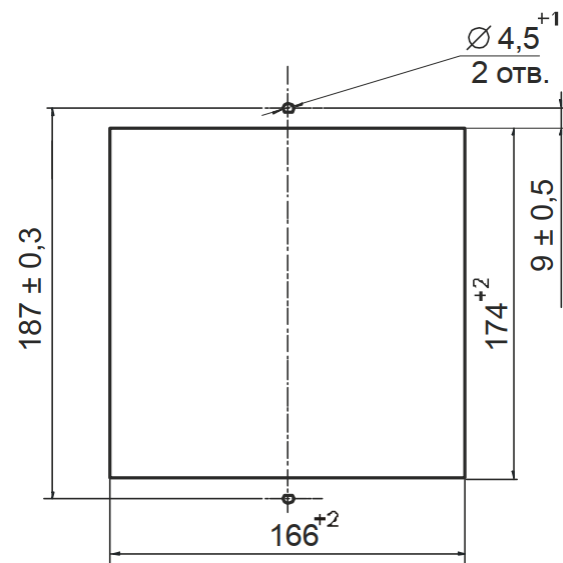
Рисунок 4 – Рекомендуемое посадочное место для установки А17
