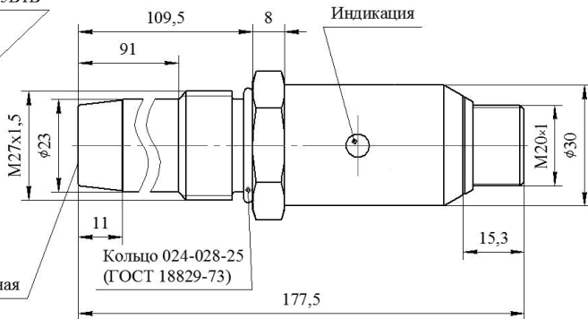
Рис.2 - Габаритный чертеж
