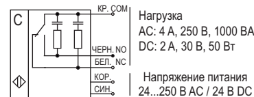
Состояние контактов реле показано при отсутствии напряжения питания
